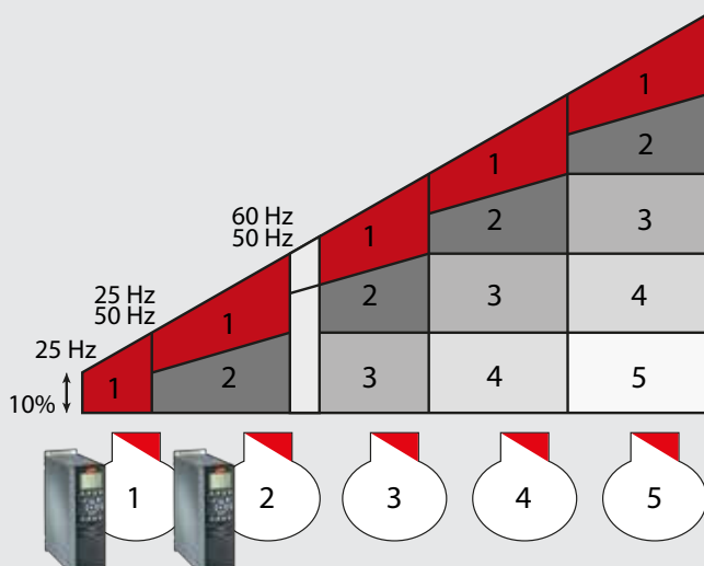
De snelheidsregeling van de hoofdcompressor plus een extra compressor zorgt voor verbeterde en gestroomlijnde ontwerp-mogelijkheden en een betere keuze van het compressorformaat voor aanpassing aan uiteenlopende 60Hz-belastingomstandigheden
