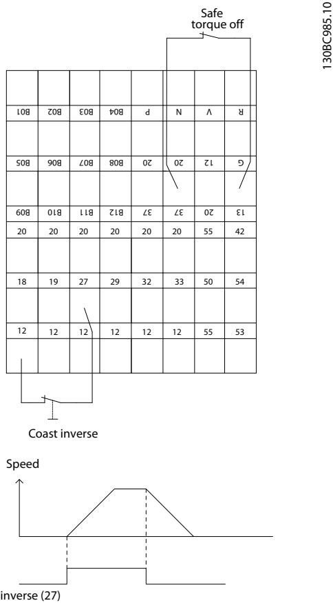
Afbeelding 3.13 Eenvoudig bedradingsvoorbeeld
