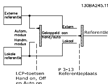
Afbeelding 4.19 Gebruik van referenties
