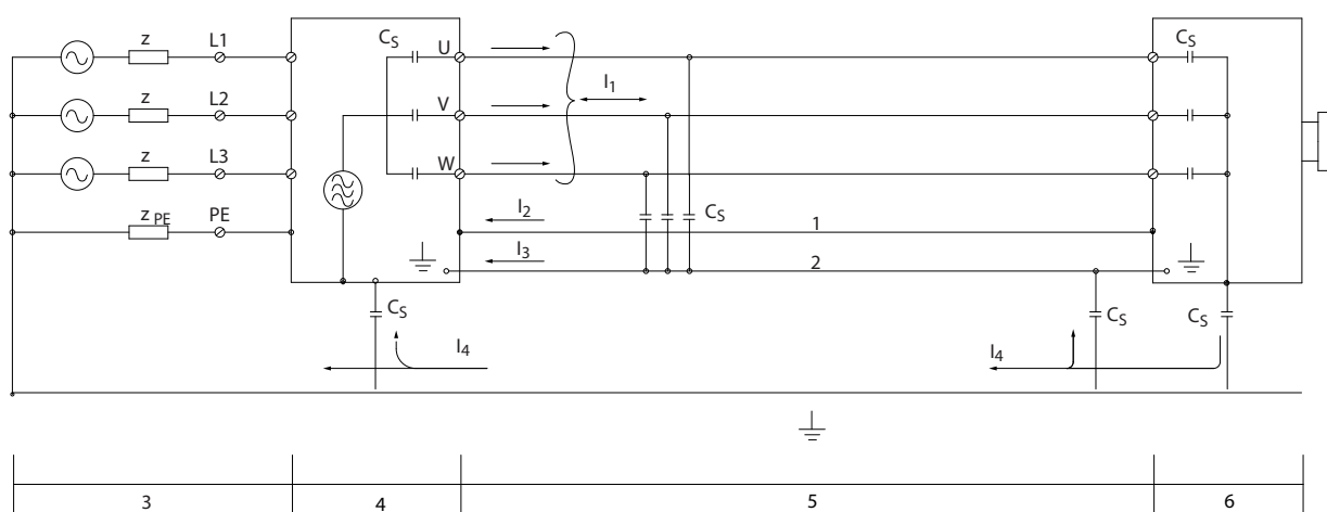
Afbeelding 2.8 Voorbeeld – lekstroom
