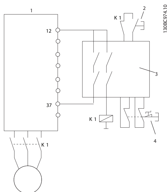
Afbeelding 4.27 Voorbeeld STO volgens stopcategorie 4
