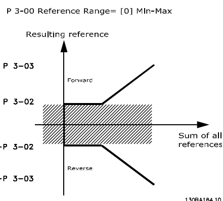
Afbeelding 2.10 Referentiebereik = [0] Min - Max
