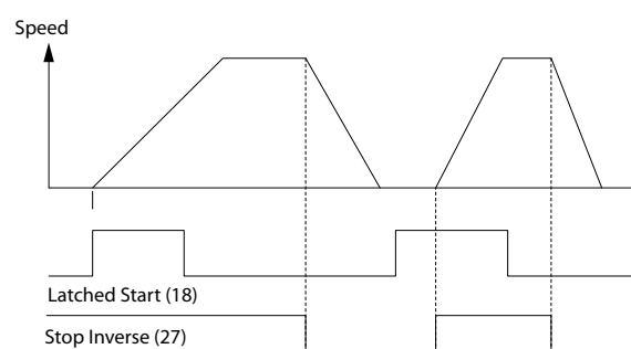
Afbeelding 4.2 Pulsstart/stop
