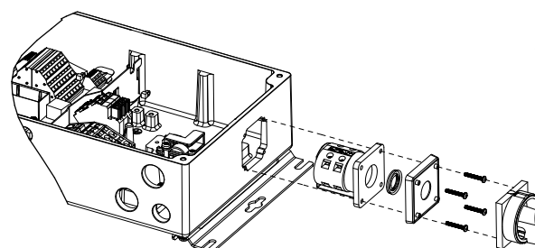
Afbeelding 3.9 Locatie van werkschakelaar, netzijde, grote eenheden (IP 66/Type 4X binnen)
