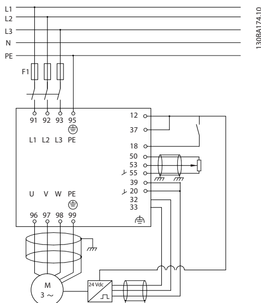
Abbeelding 4.8 Voorbeeld – aansluitingen snelheidsregeling
