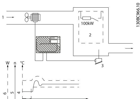
Afbeelding 4.13 Proces-PID-regeling in ventilatiesysteem
