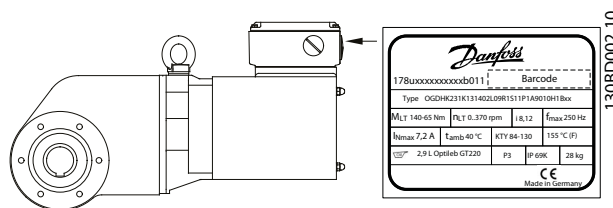
Afbeelding 3.27 Locatie motortypeplaatje
