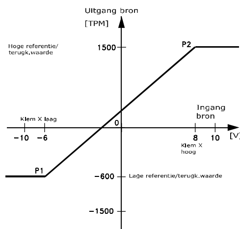
Afbeelding 2.13 Schaling van analoge en pulsreferenties en terugkoppeling
