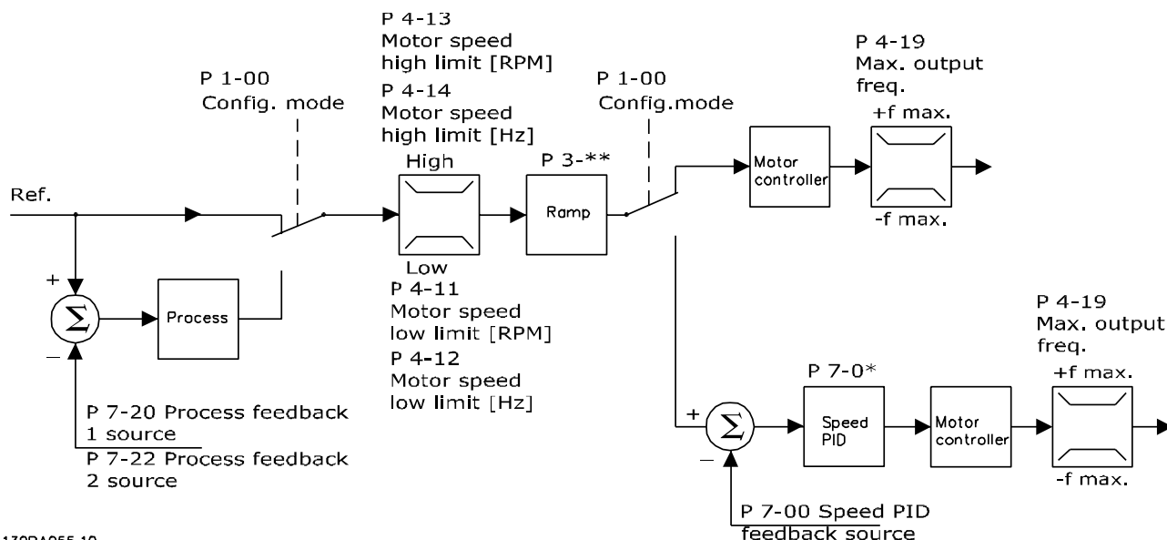
Afbeelding 4.15 Regelingsstructuur bij VVC+ in configuraties met en zonder terugkoppeling
