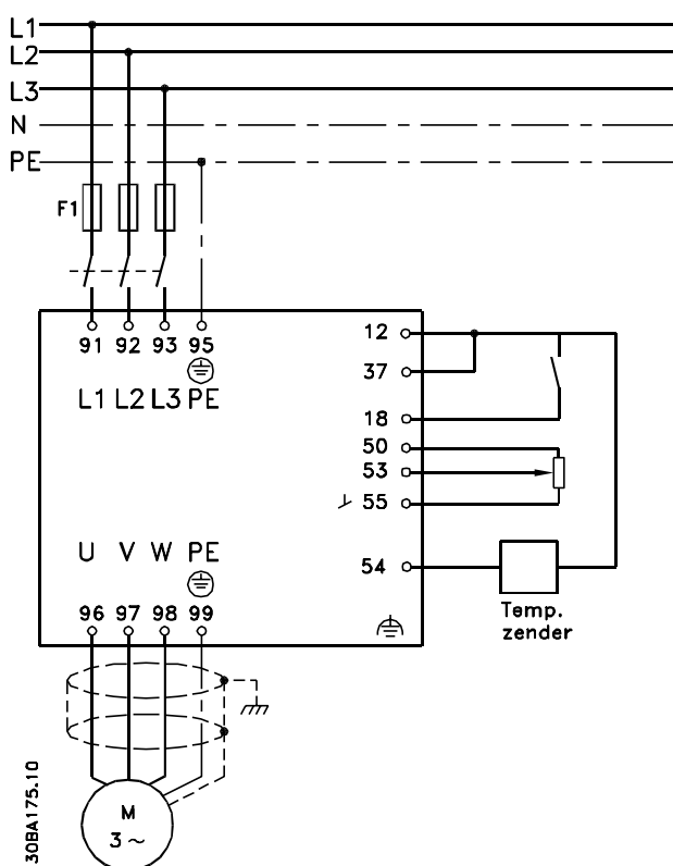
Afbeelding 3.19 Elektrisch aansluitschema
