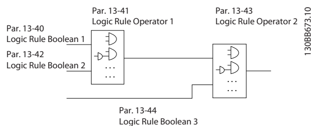
Afbeelding 2.7 Logische regels
