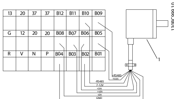
Afbeelding 5.4 Aansluitingen voor Hiperface-encoder – 2
