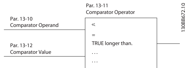
Afbeelding 2.6 Comparatoren
