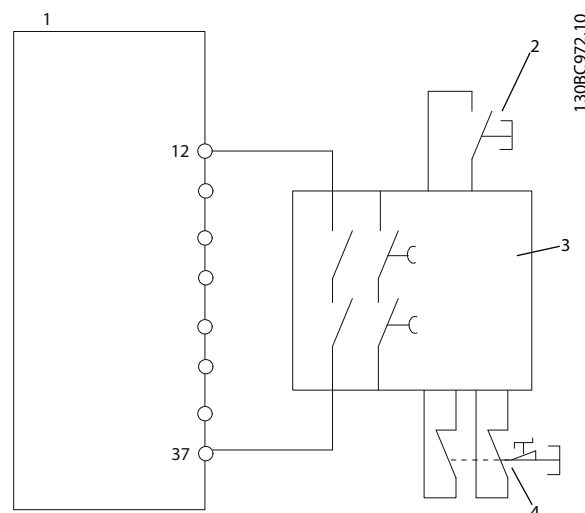
Afbeelding 4.25 Voorbeeld STO
