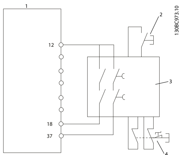
Afbeelding 4.26 Voorbeeld SS1
