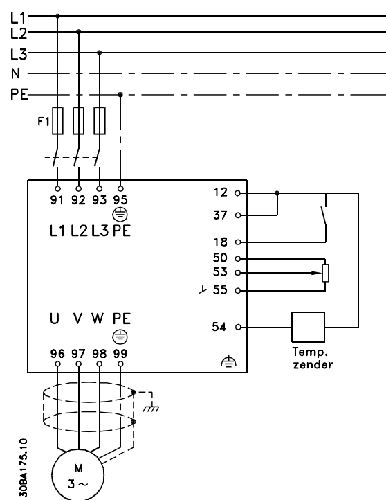
Afbeelding 4.14 Tweedraadszender
