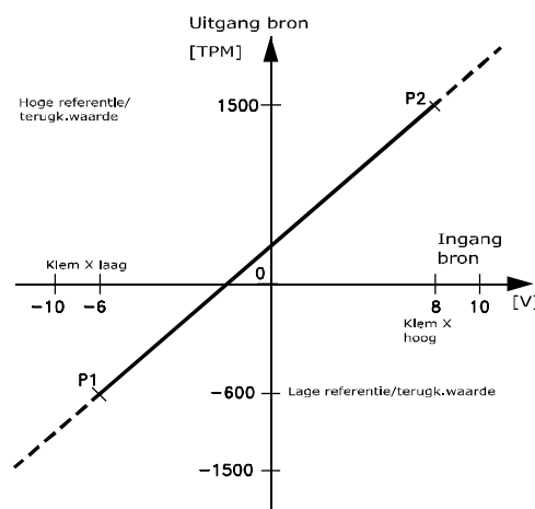
Afbeelding 2.14 Schaling referentie-uitgang
