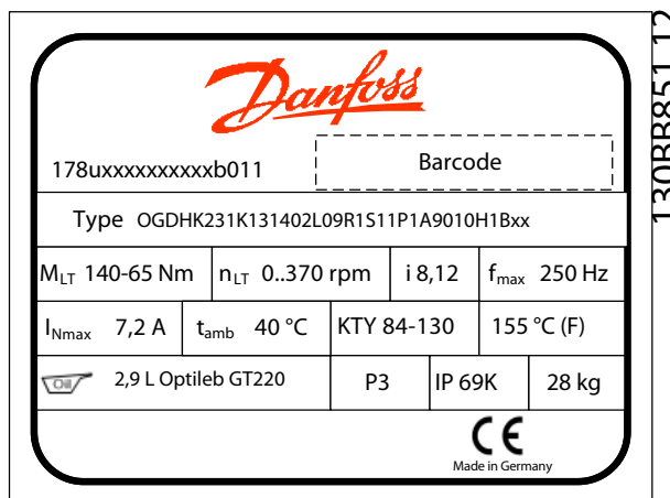
Afbeelding 3.28 Motortypeplaatje
