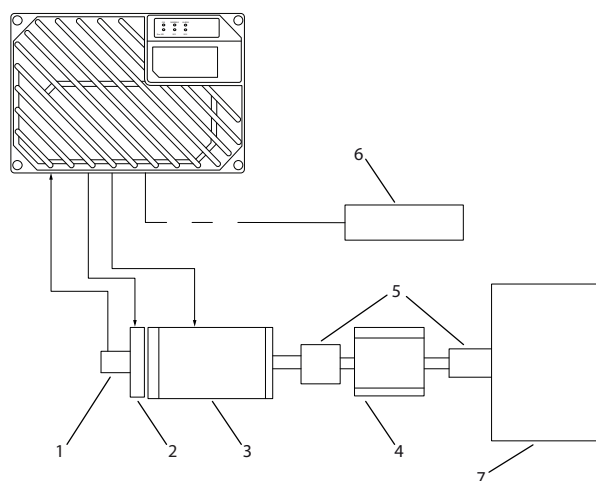
Afbeelding 4.7 Basisinstellingen voor een snelheidsregeling met terugkoppeling
