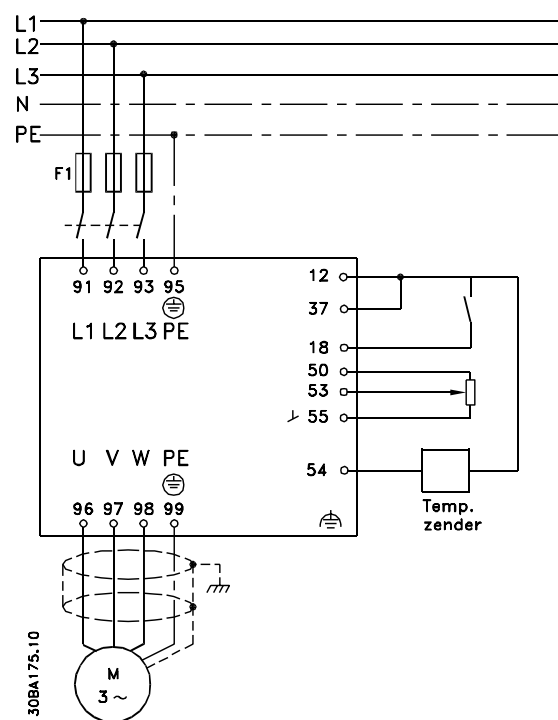
Afbeelding 4.11 Tweedraadszender
