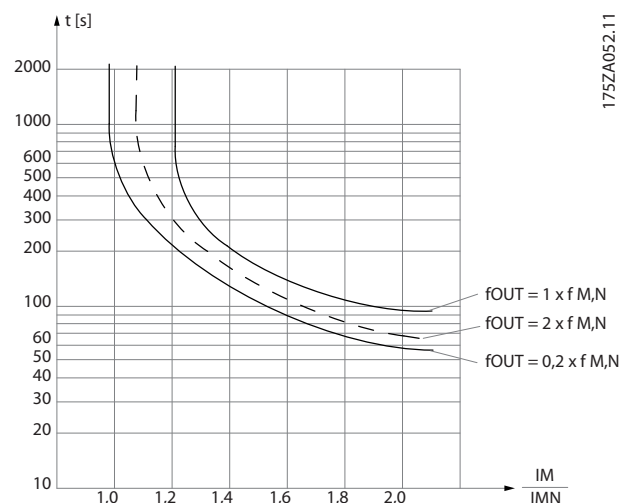
Afbeelding 3.11 ETR-functies
