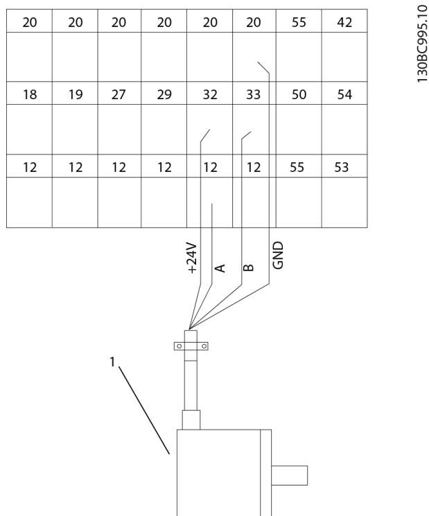
Afbeelding 4.5 Encoderaansluiting naar de frequentieomvormer
