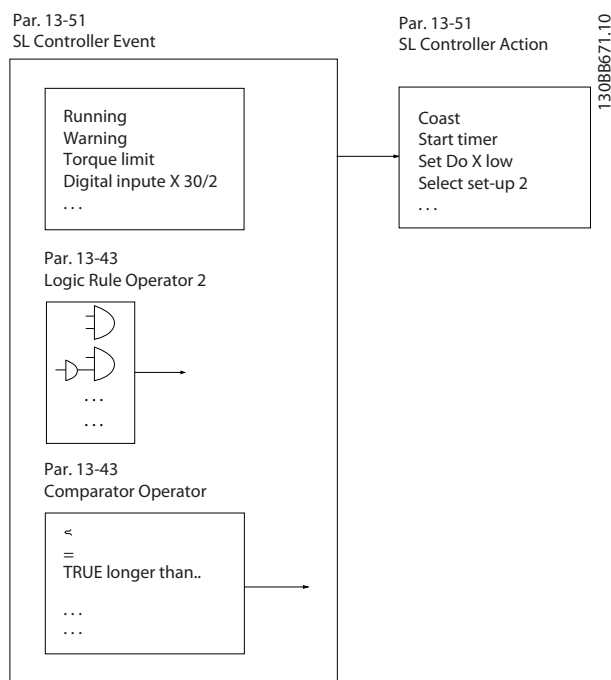
Afbeelding 2.4 Stroomregelaarstatus/gebeurtenis en actie
