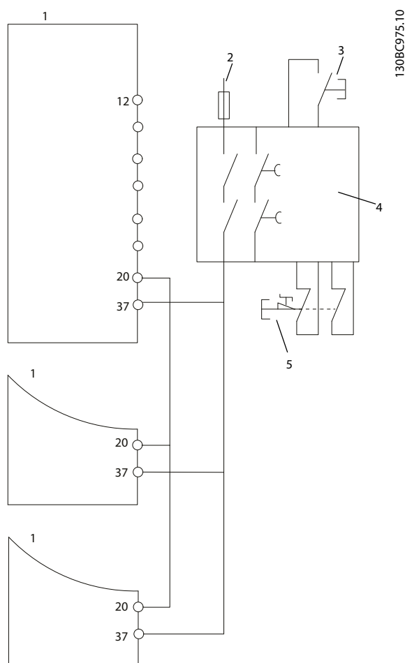
Afbeelding 4.28 Voorbeeld van parallelle aansluiting van meerdere omvormers
