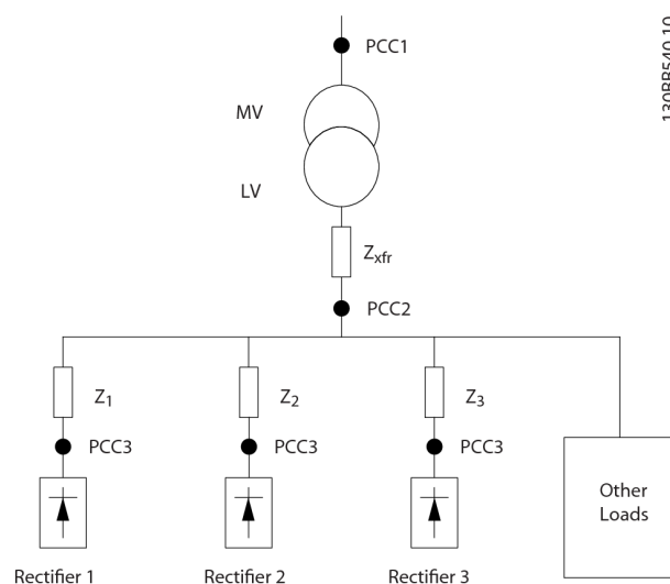
Afbeelding 3.25 Klein distributiesysteem
