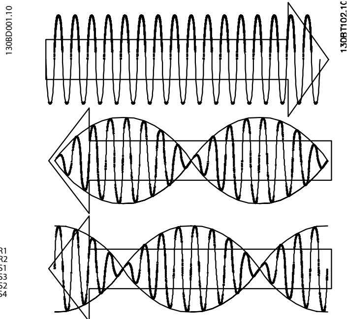
Afbeelding 5.6 Resolversignalen
