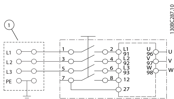
Afbeelding 3.5 Alleen voor grote eenheden: werkschakelaar aan netzijde, met doorlusklemmen
