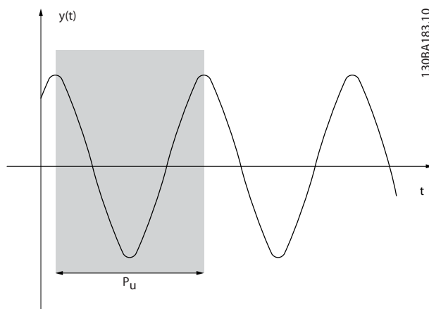
Afbeelding 4.12 Marginaal stabiel systeem
