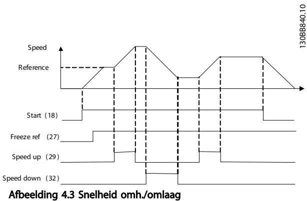
Afbeelding 4.3 Snelheid omh./omlaag
