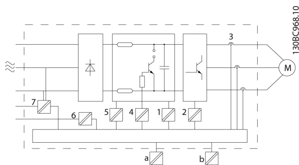
Afbeelding 2.24 Galvanische scheiding
