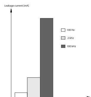
Afbeelding 2.23 Invloed van uitschakelfrequentie van de RCD
