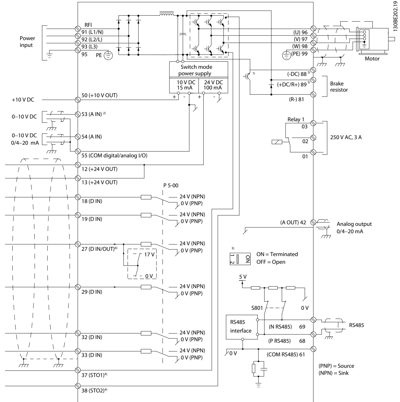
Afbeelding 4.2 Eenvoudig bedradingsschema
