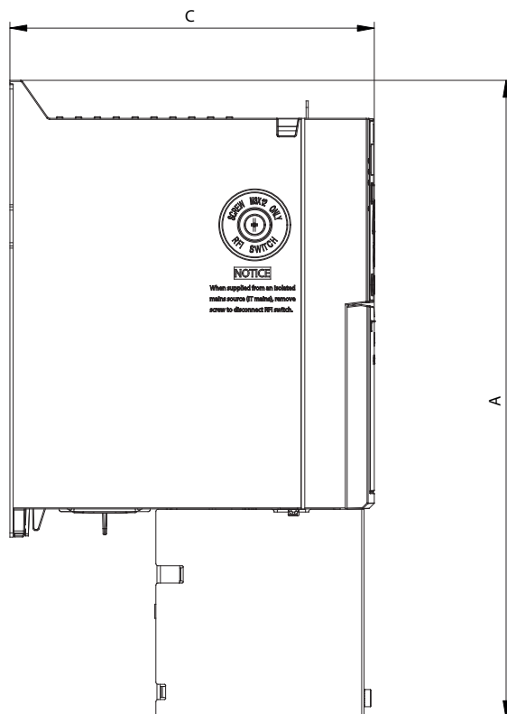
Afbeelding 9.3 Standaard met onderafdekking voor kabeldoorvoer (zonder bovenafdekking)
