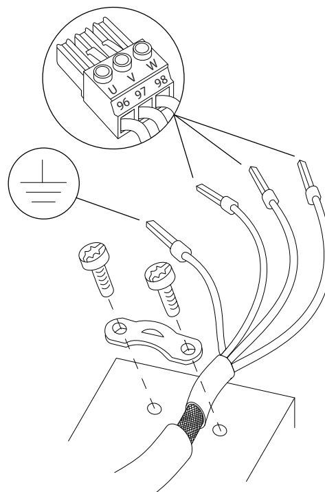
Afbeelding 4.5 Motoraansluiting
