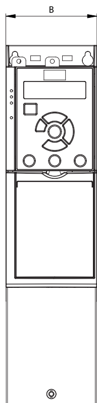
Afbeelding 9.3 Standaard met onderafdekking voor kabeldoorvoer (zonder bovenafdekking)
