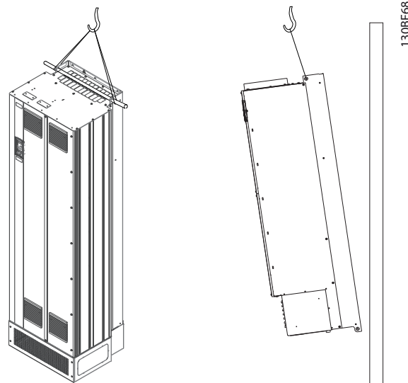
Afbeelding 4.2 Aanbevolen hijsmethode
