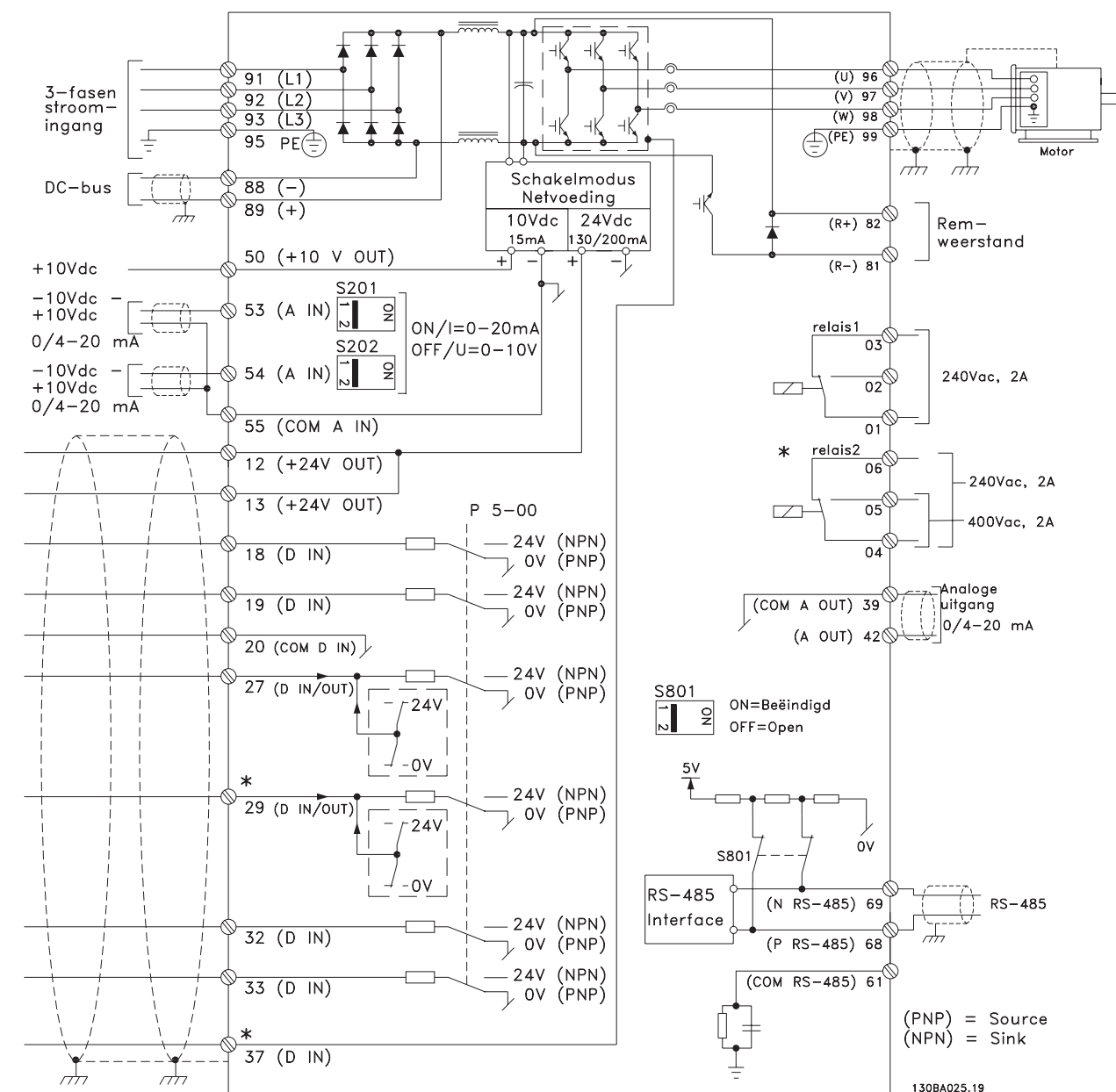
Afbeelding 5.2 Eenvoudig bedradingsschema
