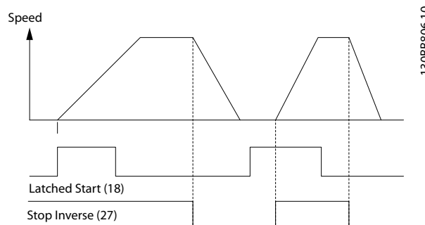
Afbeelding 8.2 Pulsstart/Stop geïnverteerd
