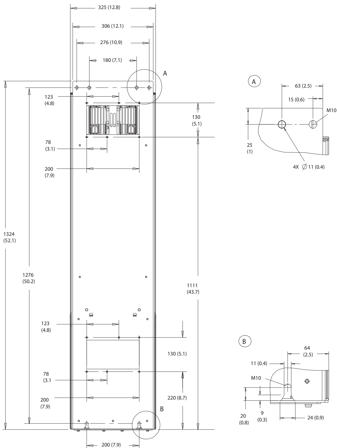
Afbeelding 10.20 Achteraanzicht D5h
