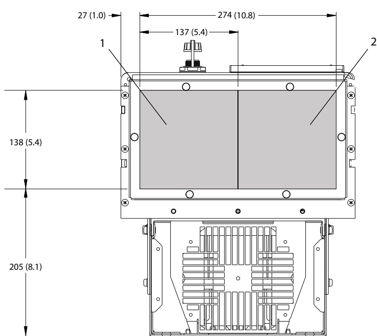
Afbeelding 10.5 Vrije ruimte bij deur voor D1h
