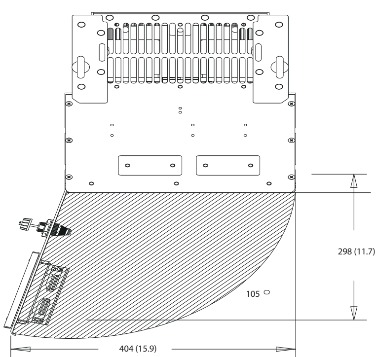
Afbeelding 10.5 Vrije ruimte bij deur voor D1h
