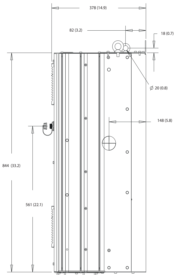
Afbeelding 10.3 Zijaanzicht D1h
