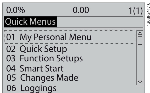
Afbeelding 3.6 Overzicht Snelmenu
