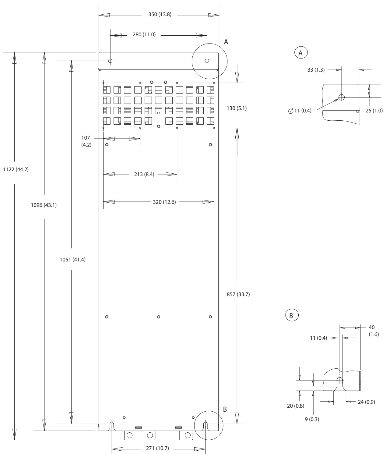
Afbeelding 10.17 Achteraanzicht D4h
