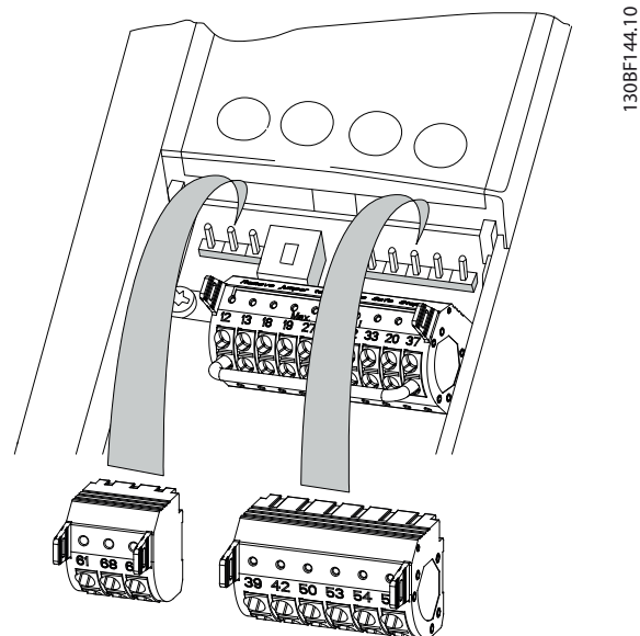
Afbeelding 5.35 Stuurklemposities
