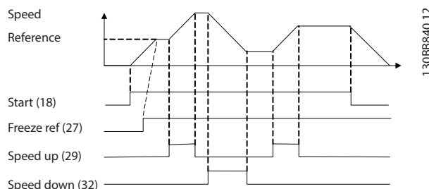
Afbeelding 8.3 Snelheid omhoog/omlaag
