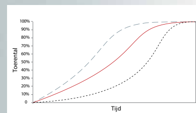
Drie Adaptive Acceleration Control (AAC) startprofielen; vroeg, constante en late acceleratie
