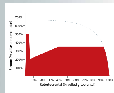
Constance stroom/stroomaanloop – hier weergegeven met kickstart
