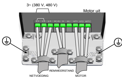
Afbeelding 12: Netvoedingaan sluitingen Vacon 20, MI4
