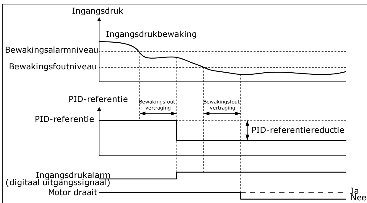
Afb. 79: De functie Ingangsdrucksdruk bewaking
