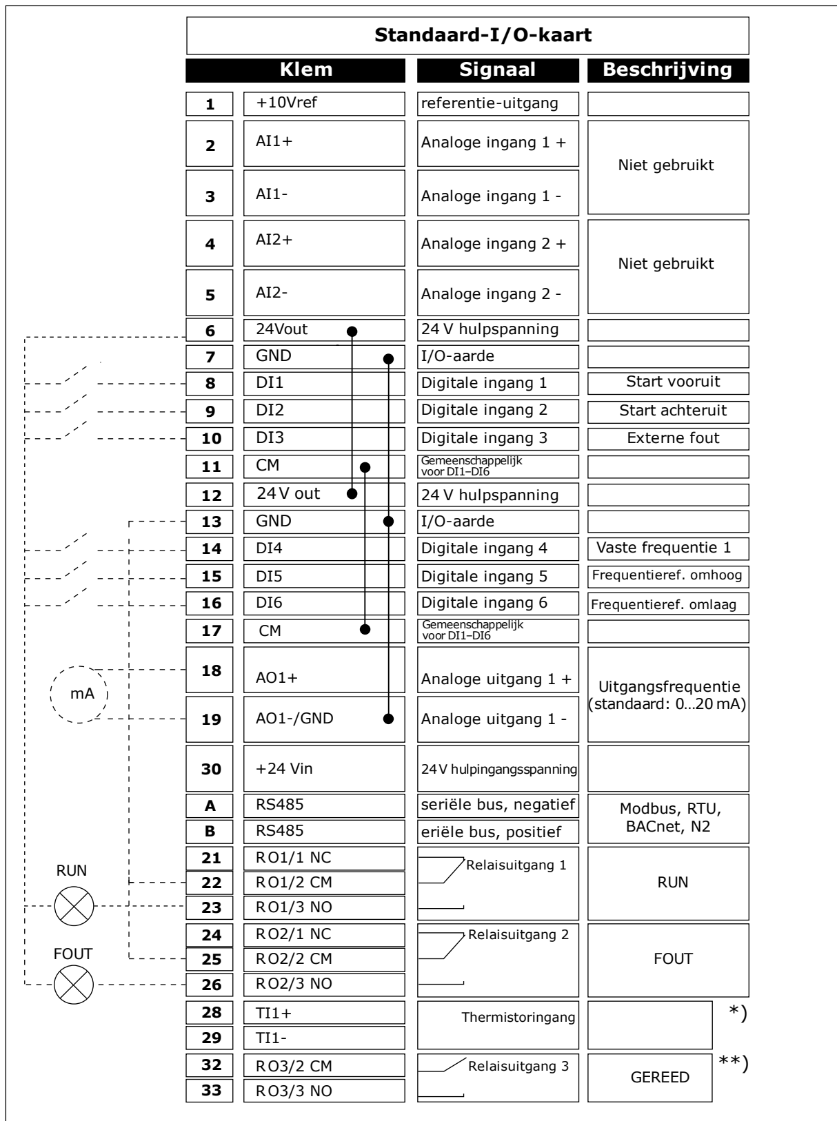
Afb. 14: De standaardaansluitingen voor besturing met de applicatie Motorpotentiometer
