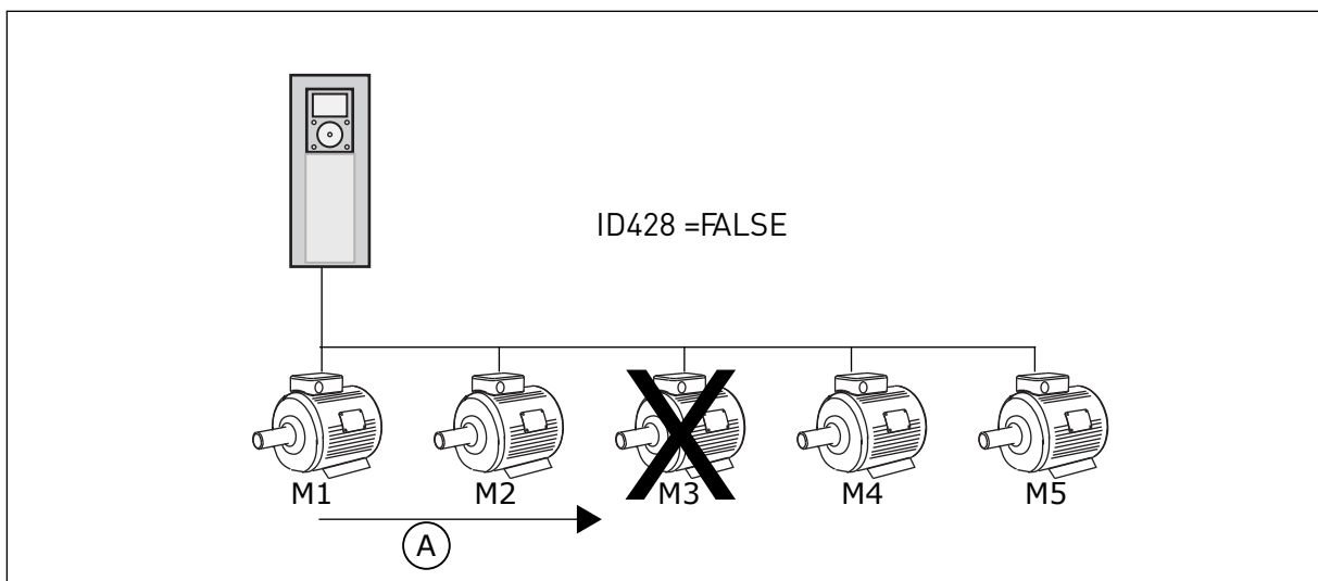
Afb. 82: Vergrendelingslogica 2
