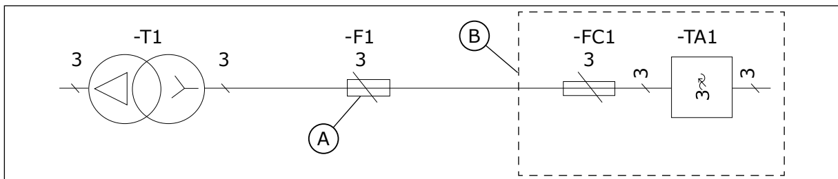
Afb. 36: Locatie van de zekeringen, MR8-MR10
