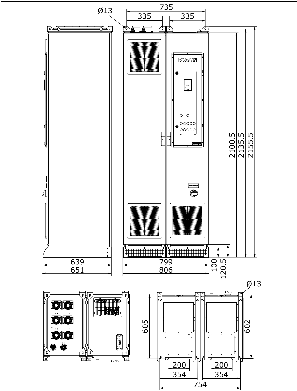
Afb. 6: De afmetingen van de kast met de optionele bekabeling via de bovenzijde, MR8, [mm], IEC
