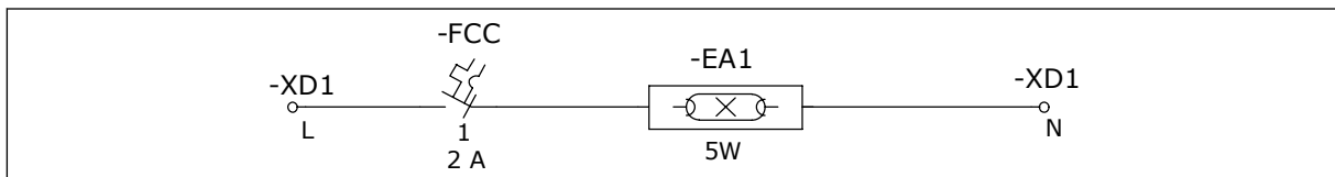
Afb. 20: De kastverlichting
