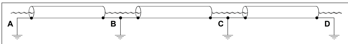
Afb. 52: Aarding in een omgeving met veel ruis en een goede potentiaalvereffening. Als de potentialen op de punten A, B, C en D sterk verschillen en niet vereffend kunnen worden, snijd de afschermingen dan door zoals aangegeven in Afb. 53.
