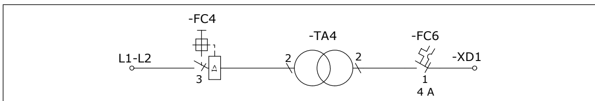
Afb. 21: De hulpspanningstransformator
