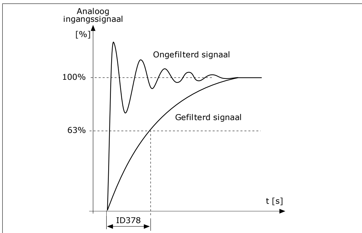
Afb. 56: Het AI1-signaalfilter
