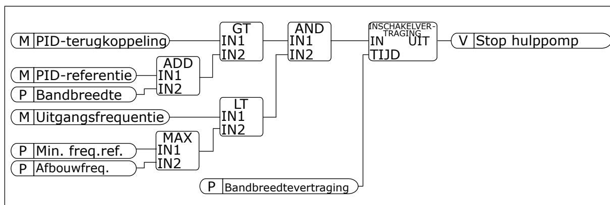
Afb. 102: Afbouwfrequentie
