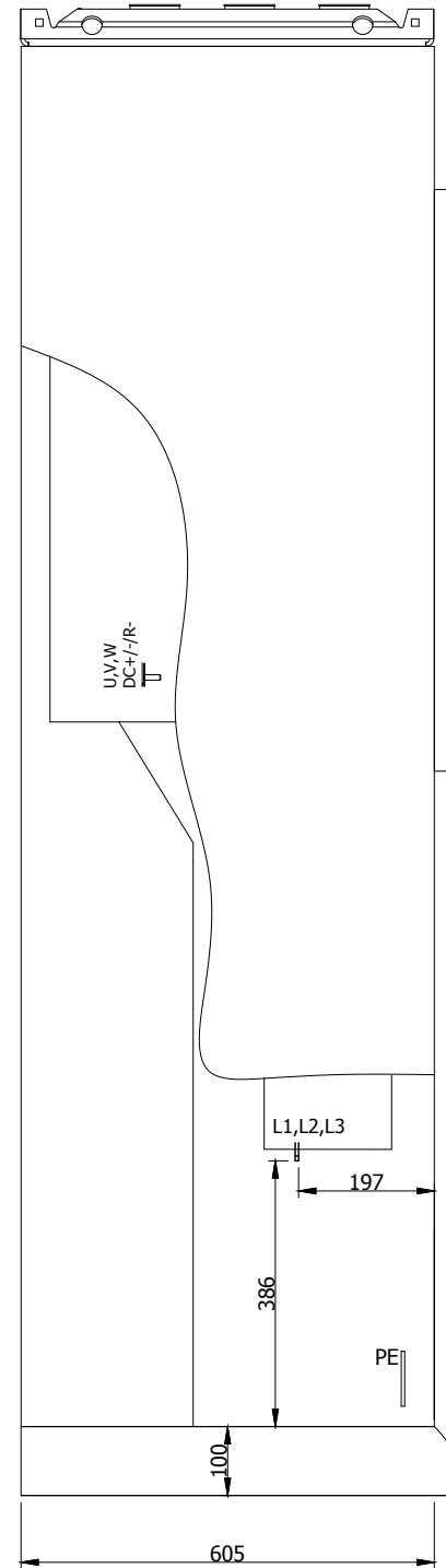
View A-A
