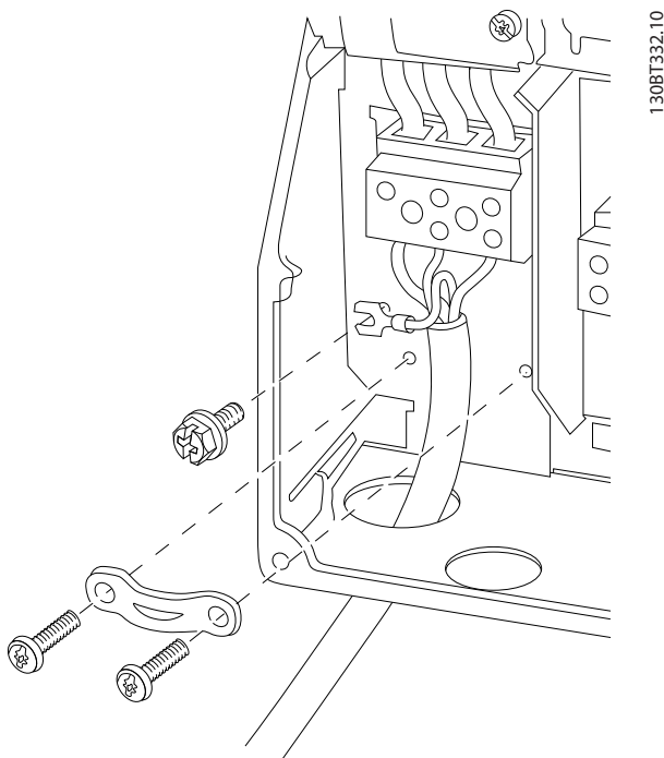
Afbeelding 9.23 Netvoeding voor behuizing B1 en B2
