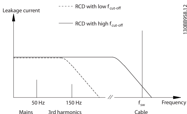
Afbeelding 9.39 Belangrijkste factoren die bijdragen aan lekstroom
