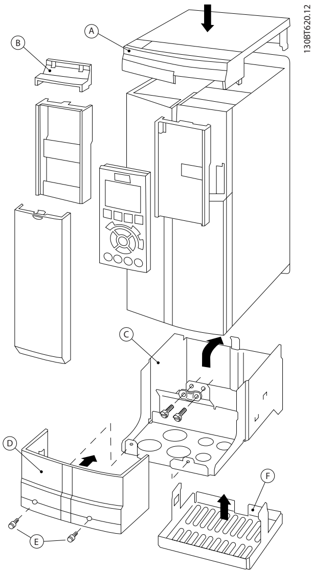
Afbeelding 11.25 Behuizingstype B3
