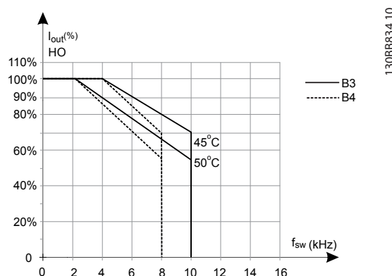
Afbeelding 6.12 Reductie van I_{out} voor diverse T_{AMB, MAX} voor behuizingstype B3 en B4, bij gebruik van SFAVM en een hoge overbelastingsmodus (overbelastingskoppel van 160%)
