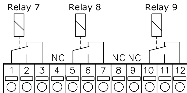
Afbeelding 11.10 Relais
