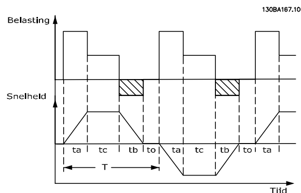
Afbeelding 5.8 Typische remcyclus
