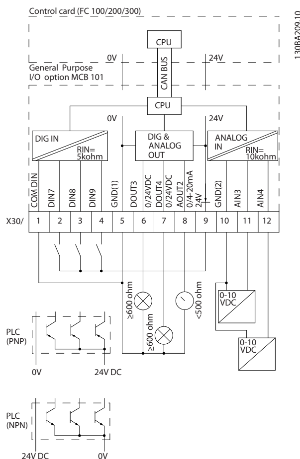
Afbeelding 11.2 Principeschema
