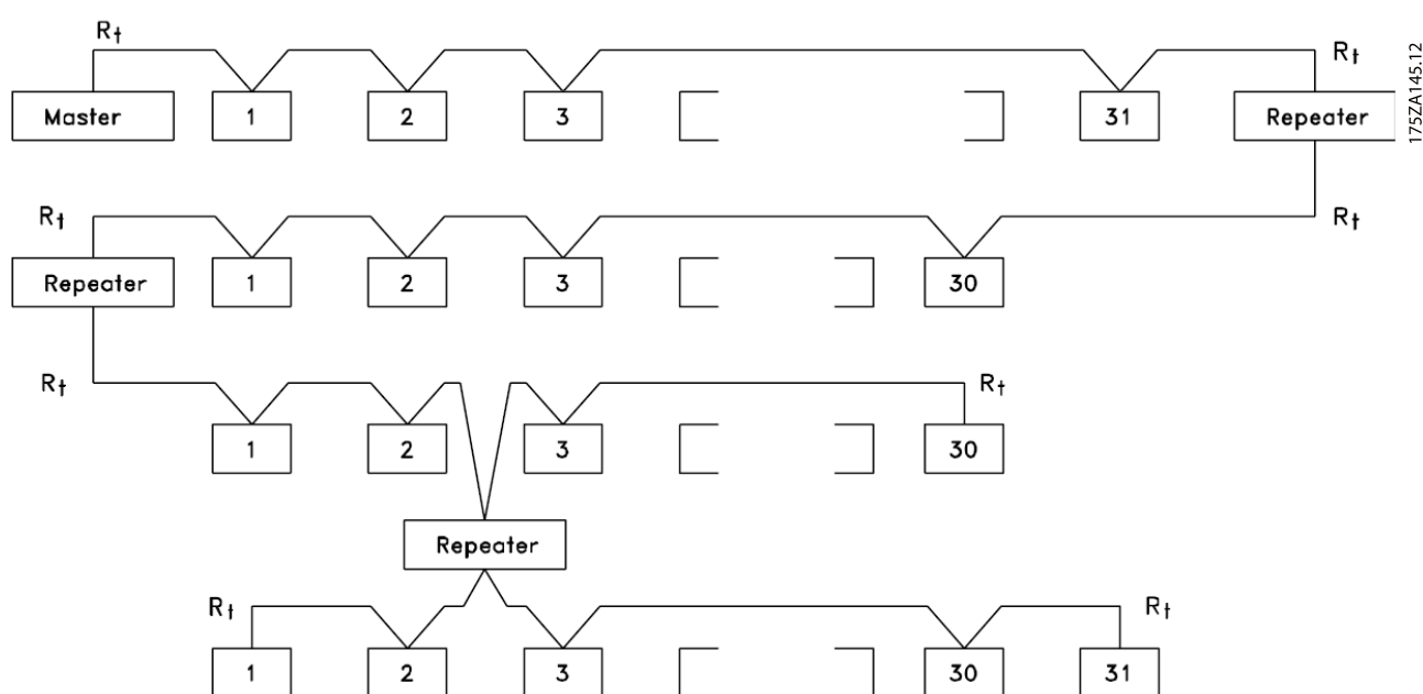
Afbeelding 12.1 RS-485-businterface
