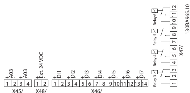
Abbeelding 11.17 Elektrische aansluitingen voor MCB 113
