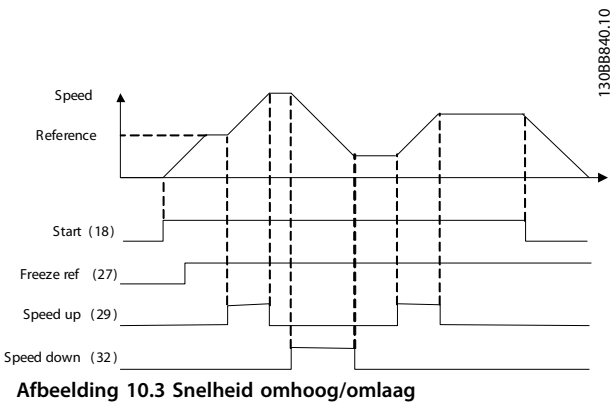
Afbeelding 10.3 Snelheid omhoog/omlaag
