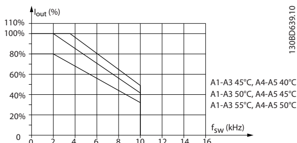
Afbeelding 6.3 Reductie van I_{out} voor diverse T_{AMB, MAX} voor behuizingstype A, bij gebruik van SFAVM
