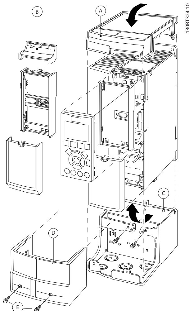
Afbeelding 11.24 Behuizingstype A3
