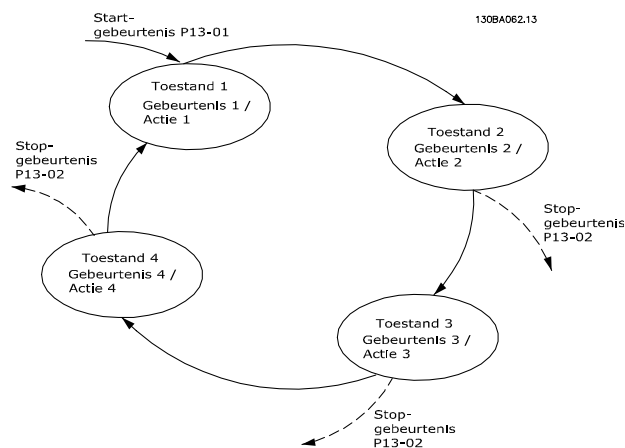
Afbeelding 4.5 Volgorde van uitvoering wanneer 4 gebeurtenissen/acties zijn geprogrammeerd
