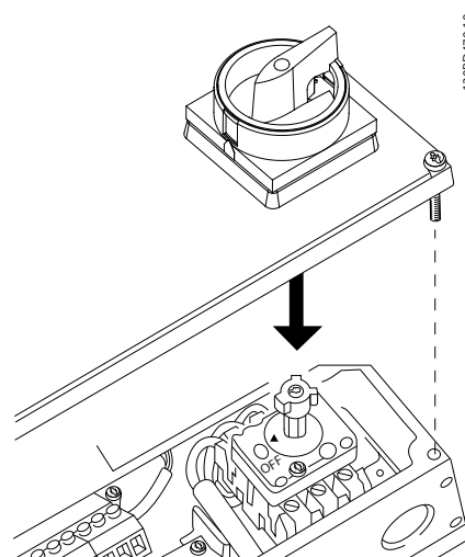
Afbeelding 9.45 Positie van netschakelaar
