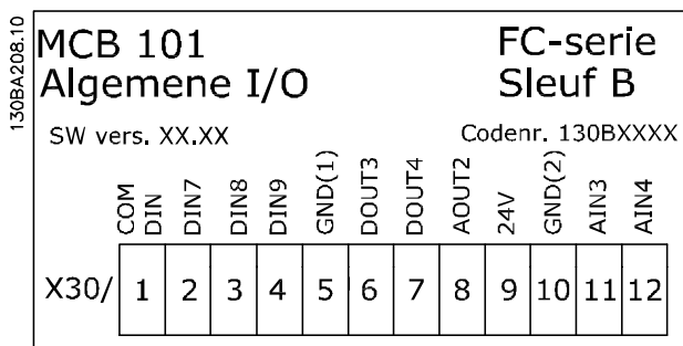
Afbeelding 11.1 Optie MCB 101
