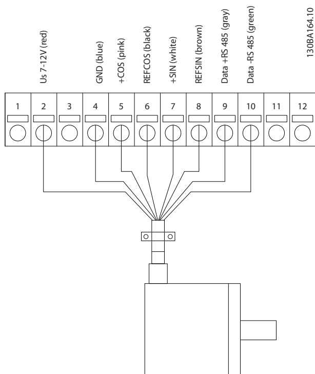
Afbeelding 11.4 SinCos-encoder Hiperface
