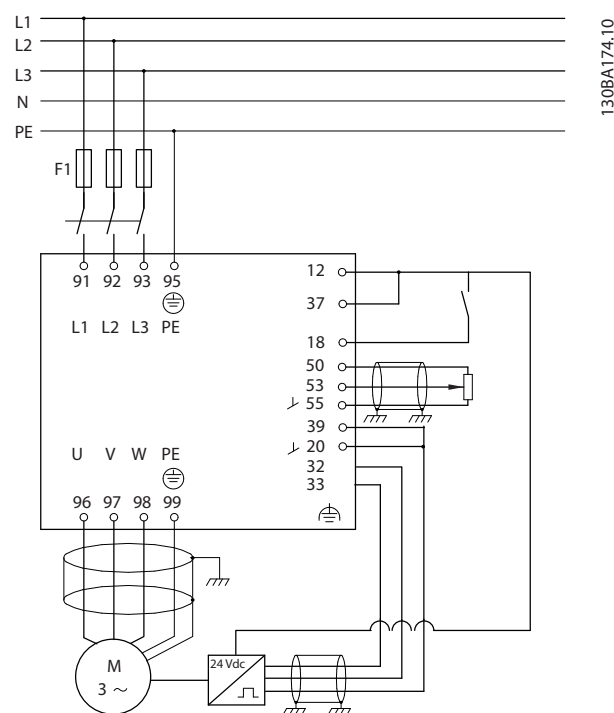
Afbeelding 10.7 Voorbeeld – aansluitingen snelheidsregeling
