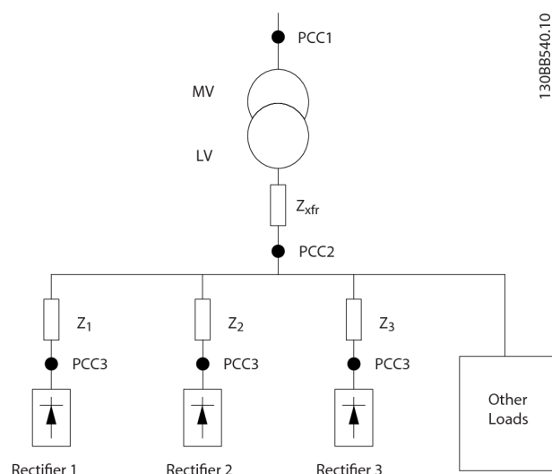
Afbeelding 5.5 Klein distributiesysteem
