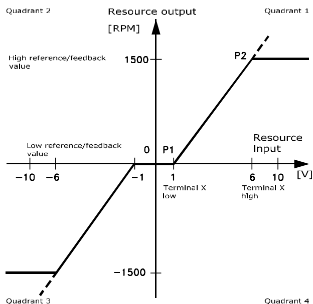
Afbeelding 3.19 Dode band
