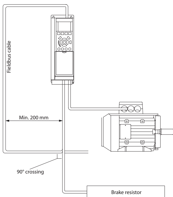
Afbeelding 12.4 Bekabeling
