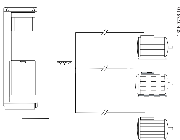
Afbeelding 9.54 LC-filter voor lange parallelle kabels
