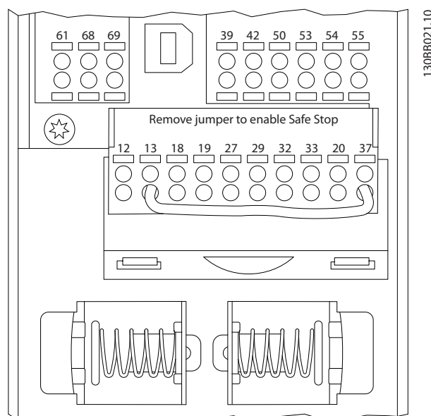
Afbeelding 12.3 Stuurkaartklemmen
