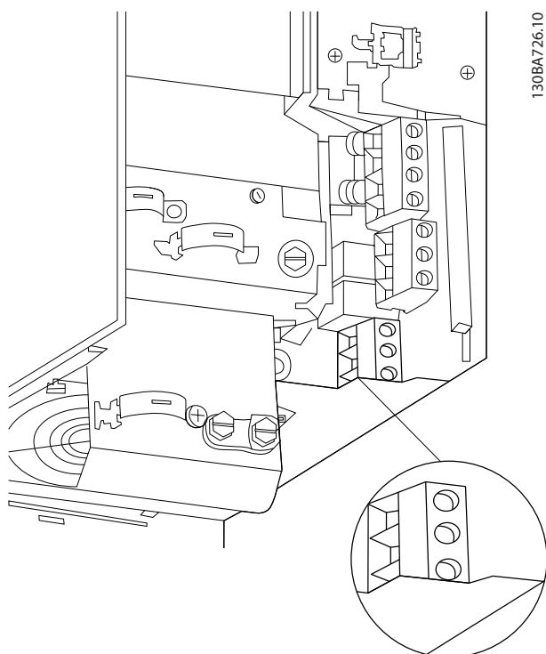
Afbeelding 9.33 Motoraansluiting voor behuizing B3
