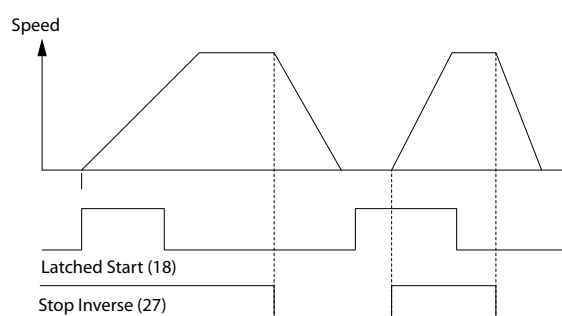
Afbeelding 10.2 Pulsstart/Stop geïnverteerd
