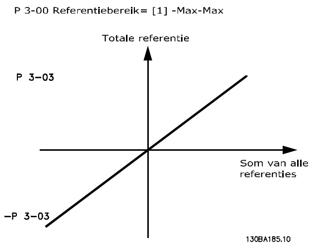
Afbeelding 3.15 Totale referentie
