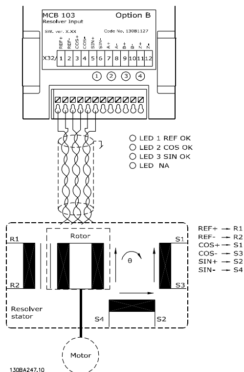
Afbeelding 11.6 MCB 103-resolveringang
