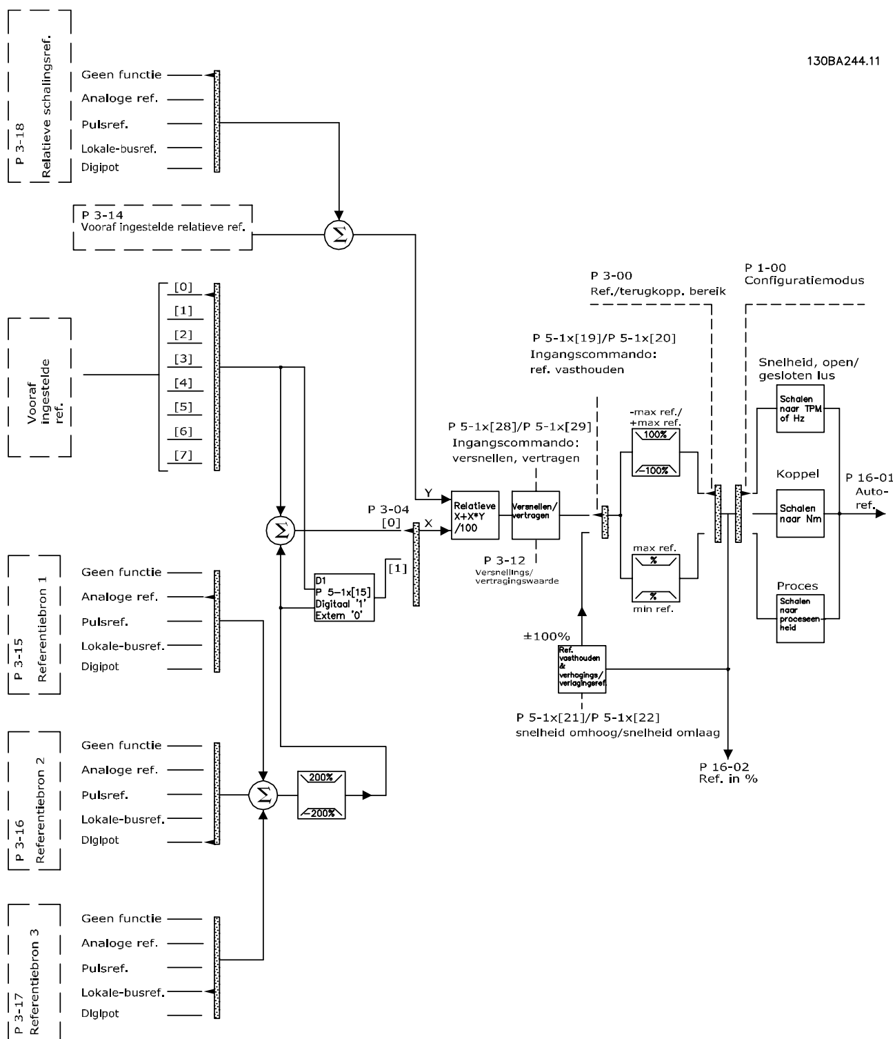
Afbeelding 3.13 Externe referentie
