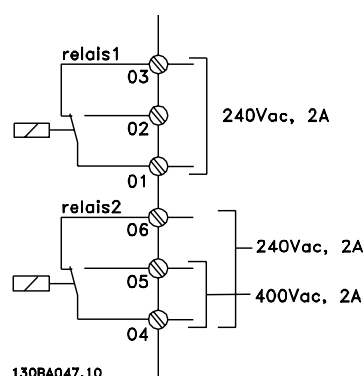
Afbeelding 9.41 Relaisuitgang 1 en 2
