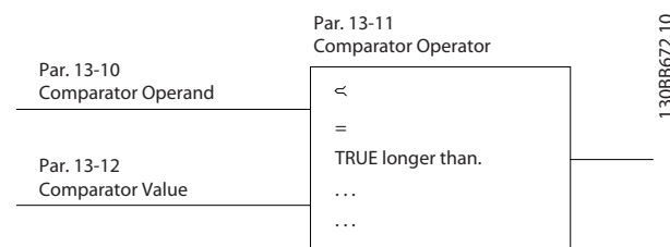
Afbeelding 4.6 Comparatoren
