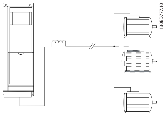
Afbeelding 9.53 Parallele kabels met belasting
