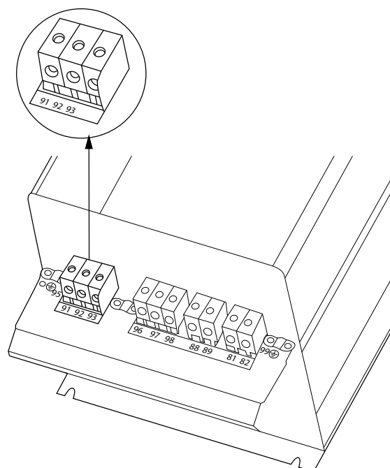
Afbeelding 9.27 Netvoeding voor behuizing C3 (IP 20)
