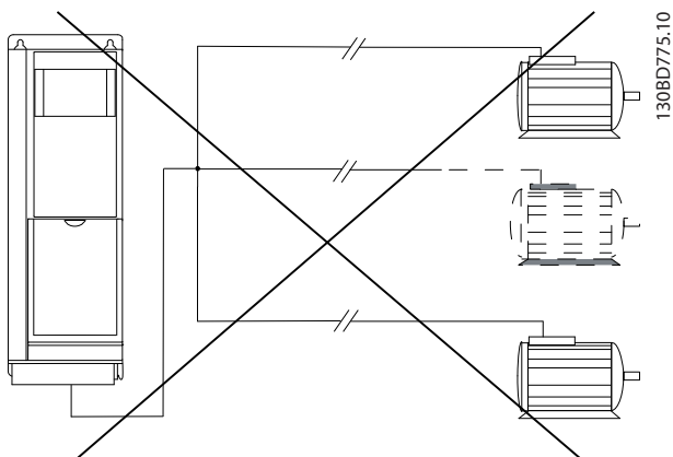
Afbeelding 9.51 Gemeenschappelijk aansluitpunt voor lange kabellengtes
