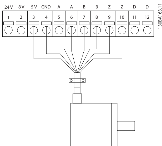
Afbeelding 11.3 Incrementele encoder
