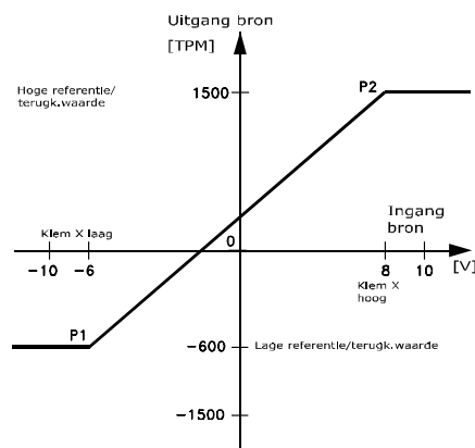
Afbeelding 3.17 Schaling van analoge en pulsreferenties en terugkoppeling
