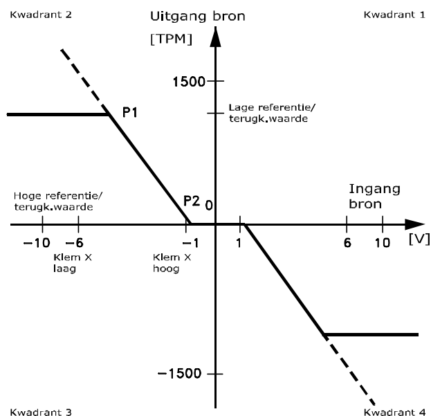
Afbeelding 3.20 Omgekeerde dode band
