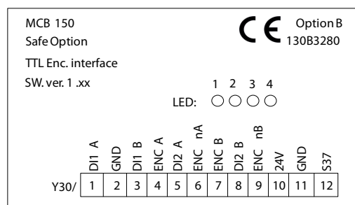
Afbeelding 11.20 MCB 150
