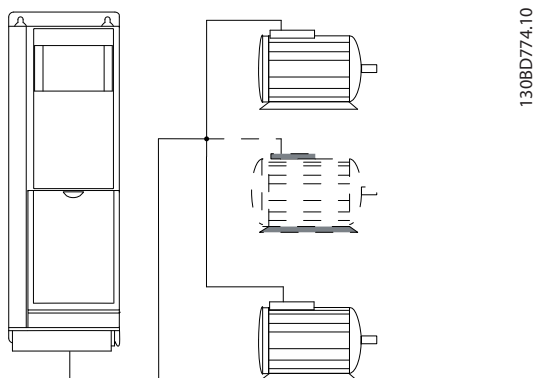
Afbeelding 9.50 Gemeenschappelijk aansluitpunt voor korte kabellengtes
