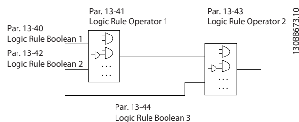
Afbeelding 4.7 Log. regels
