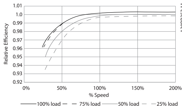
Afbeelding 6.35 Typische rendementscurves
