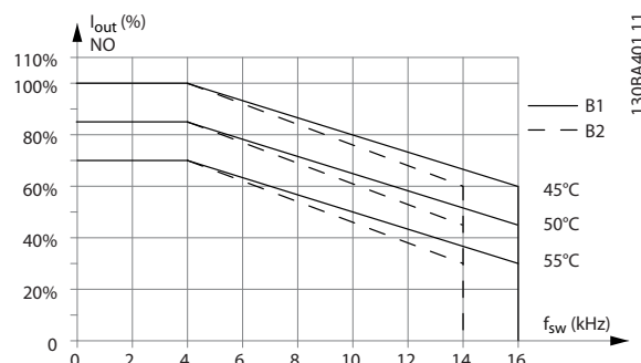
Afbeelding 6.7 Reductie van I_{out} voor diverse T_{AMB, MAX} voor behuizingstype B1 en B2, bij gebruik van 60° AVM en een normale overbelastingsmodus (overbelastingskoppel van 110%)
