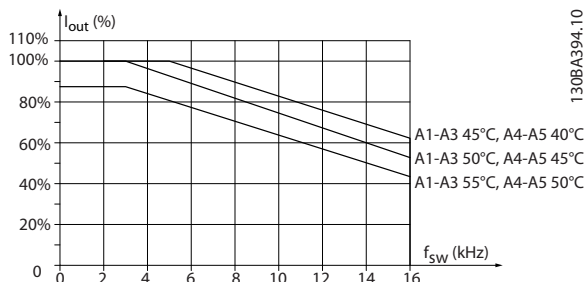
Afbeelding 6.4 Reductie van I_{out} voor diverse T_{AMB, MAX} voor behuizingstype A, bij gebruik van 60° AVM en een motorkabel van maximaal 10 m
