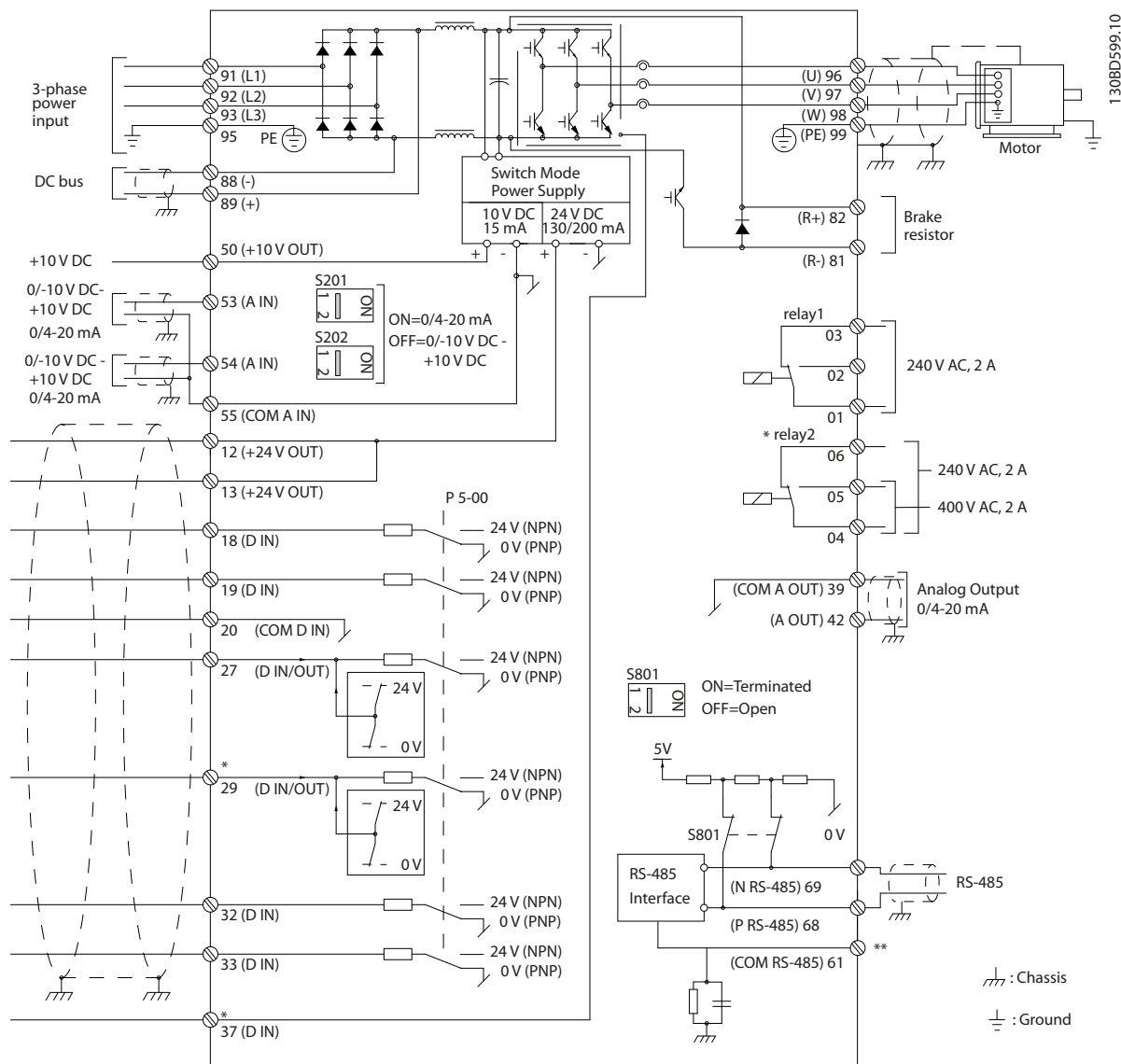
Afbeelding 3.2 Eenvoudig bedradingsschema
