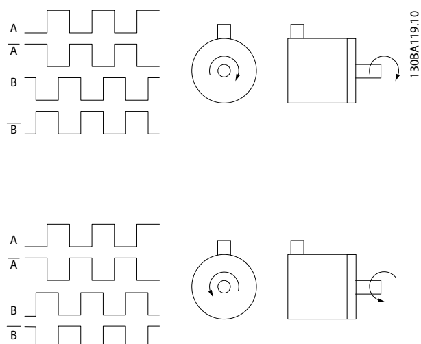
Afbeelding 11.5 Draairichting
