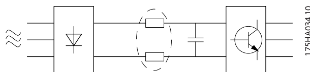
Afbeelding 5.4 Tussenkringspoelen
