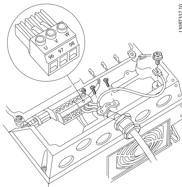
Afbeelding 9.31 Motoraansluiting voor behuizing A4/A5
