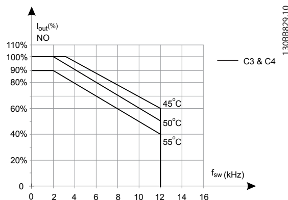
Afbeelding 6.23 Reductie van I_{out} voor diverse T_{AMB, MAX} voor behuizingstype C3 en C4, bij gebruik van 60° AVM en een normale overbelastingsmodus (overbelastingskoppel van 110%)
