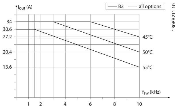
Afbeelding 6.18 Reductie van de uitgangsstroom wegens schakelfrequentie en omgevingstemperatuur voor behuizingstype B2 en B4, 60° AVM. NB De grafiek gaat uit van de stroom als absolute waarde en geldt voor zowel een hoge als een normale overbelasting.
