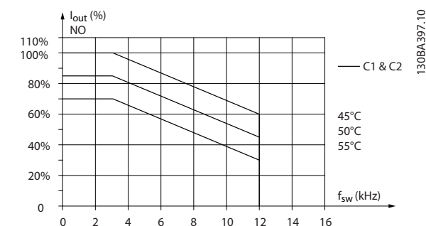
Afbeelding 6.21 Reductie van I_{out} voor diverse T_{AMB, MAX} voor behuizingstype C1 en C2, bij gebruik van 60° AVM en een normale overbelastingsmodus (overbelastingskoppel van 110%)
