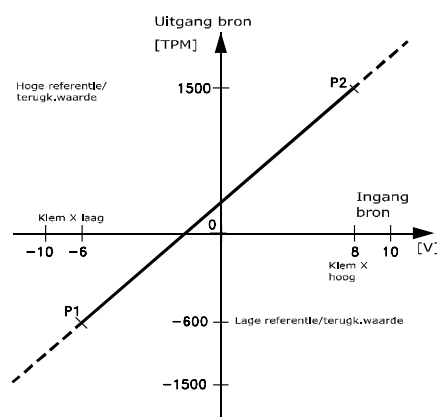
Afbeelding 3.18 Schaling referentie-uitgang
