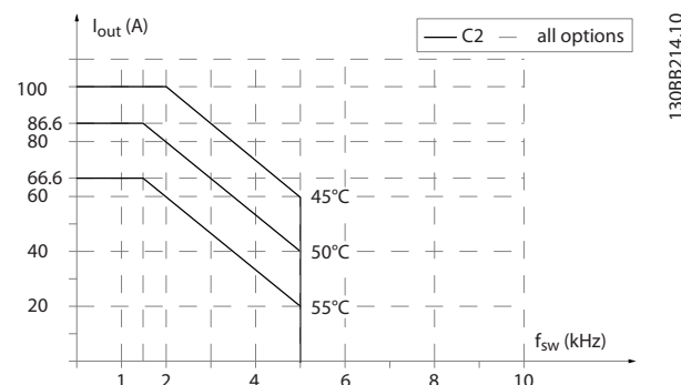
Afbeelding 6.33 Reductie van de uitgangsstroom wegens schakelfrequentie en omgevingstemperatuur voor behuizingstype C2, SFAVM. NB De grafiek gaat uit van de stroom als absolute waarde en geldt voor zowel een hoge als een normale overbelasting.
