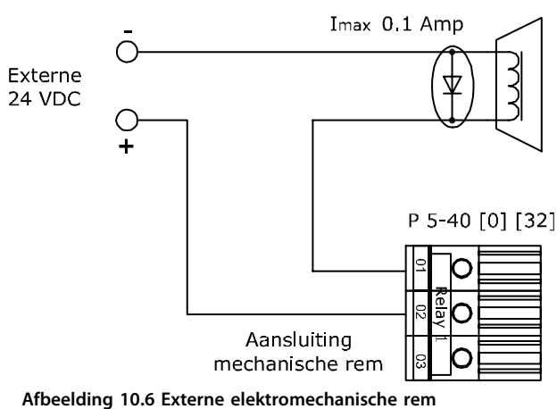
Afbeelding 10.6 Externe elektromechanische rem
