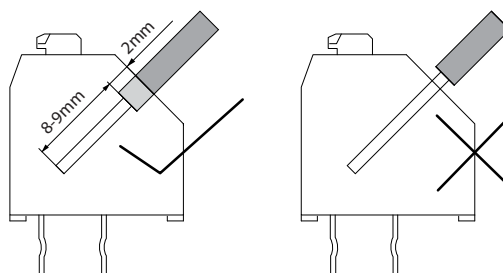
Afbeelding 11.11 Juiste kabeldoorvoer
