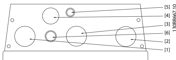
Afbeelding 9.7 B1 – IP 21
