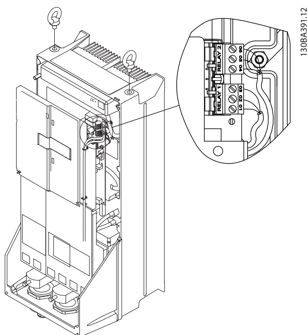
Afbeelding 9.43 Klemmen voor relaisaansluiting (behuizingstype C1 en C2).
