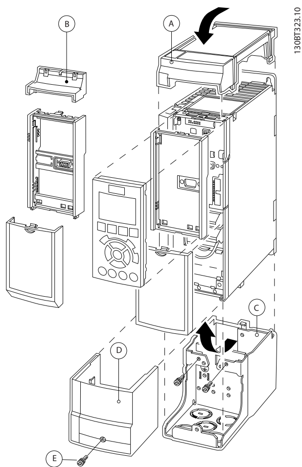
Afbeelding 11.23 Behuizingstype A2
