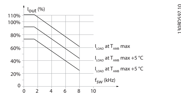
Afbeelding 6.34 Reductie van de uitgangsstroom wegens schakelfrequentie en omgevingstemperatuur voor behuizingstype C3
