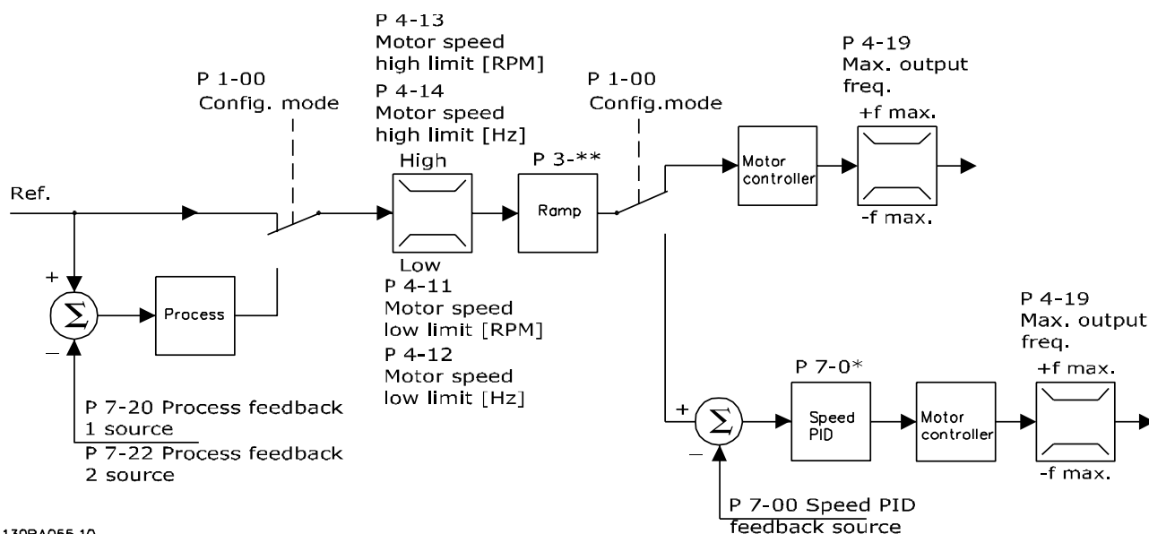
Afbeelding 3.6 Regelstructuur op basis van VVC plus in configuraties met en zonder terugkoppeling
