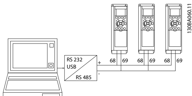
Afbeelding 12.2 Parallelle aansluitingen
