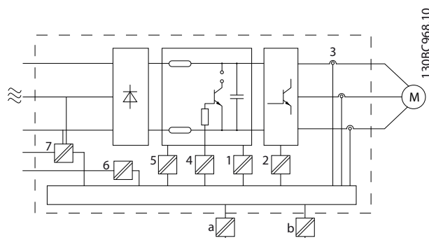
Afbeelding 5.7 Galvanische scheiding
