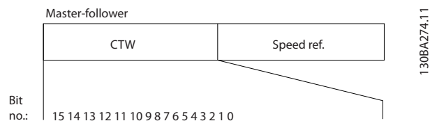
Afbeelding 12.16 Stuurwoord
