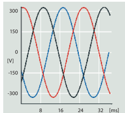
Geoptimaliseerde harmonische prestaties Efficiënte harmonischedreductie beschermt de elektronica en verhoogt het rendement.
