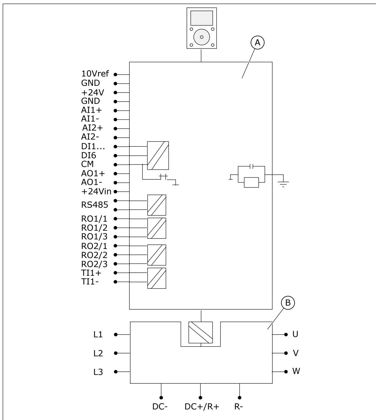
Afb. 45: Galvanische isolatie
