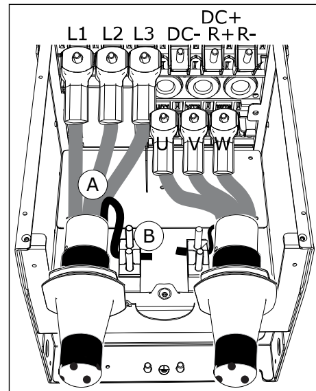
A. Aansluiting van de kabels B. Aardaansluiting van MR8
