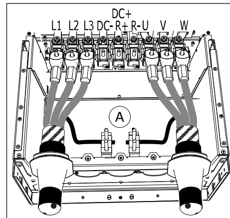
A. Aardaansluiting van MR9
