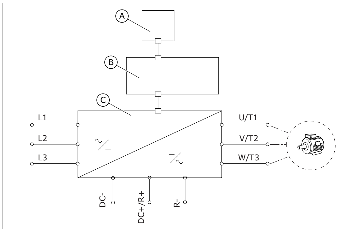
Afb. 35: Principeschema aansluitingen
