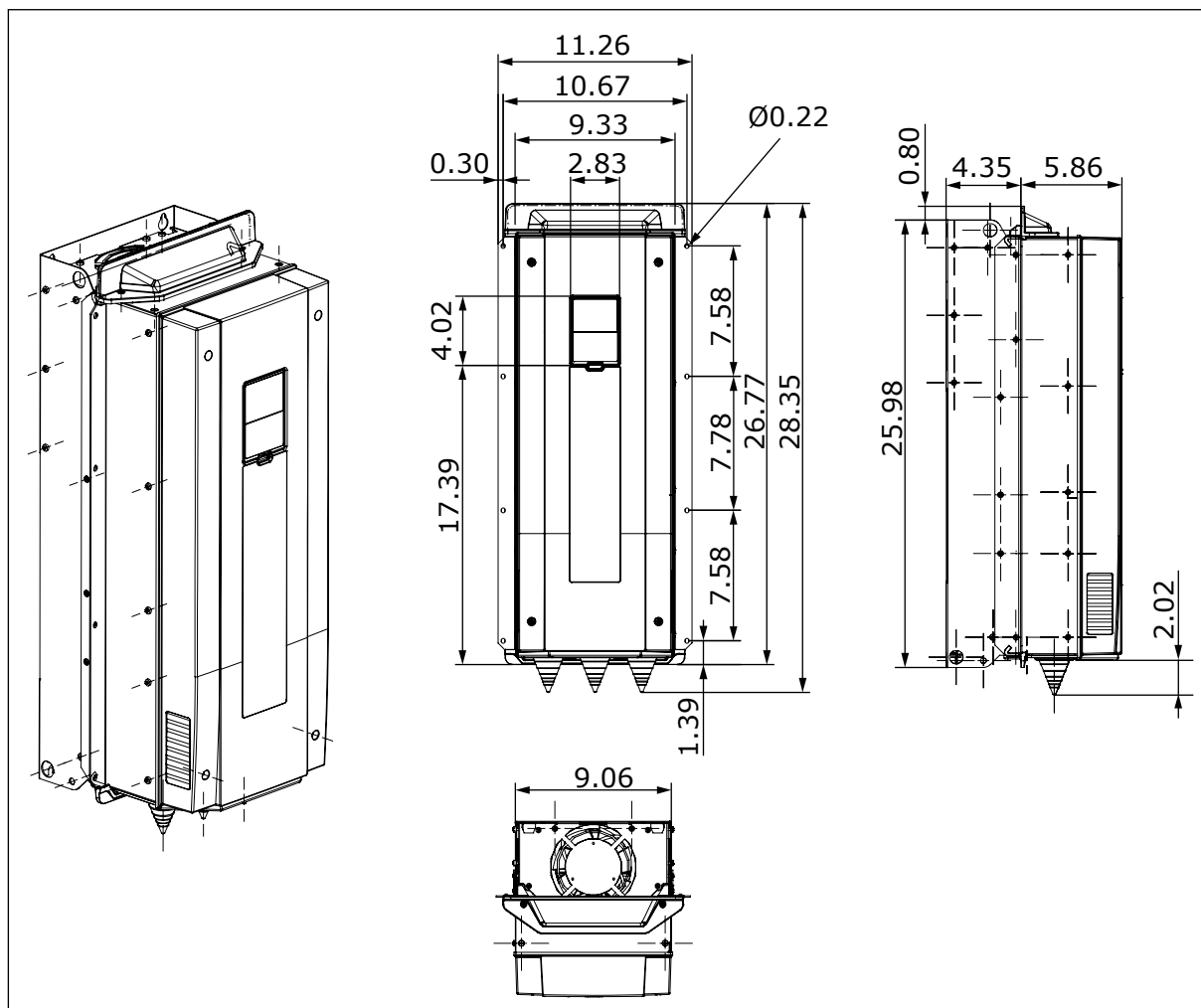
Afb. 30: Maten van de AC-frequentieregelaar, wartelplaatmontage, MR7 [inch]
