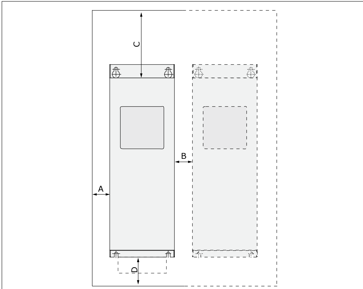
Afb. 33: Ruimte voor installatie
